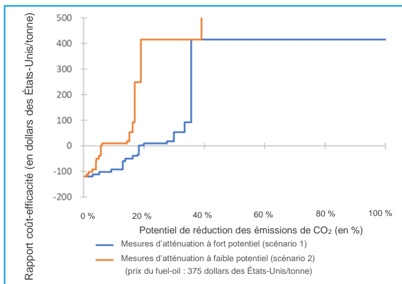
Figure 25 - Courbe des coûts de réduction marginaux pour 2050
